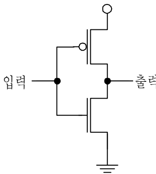
(e) 트랜지스터 회로도
